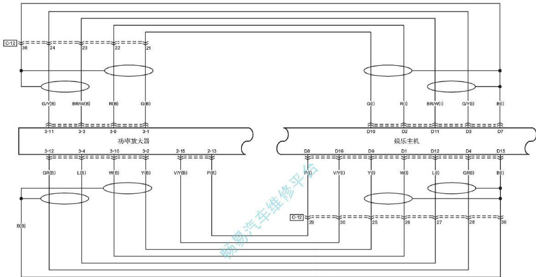
功率放大器2
